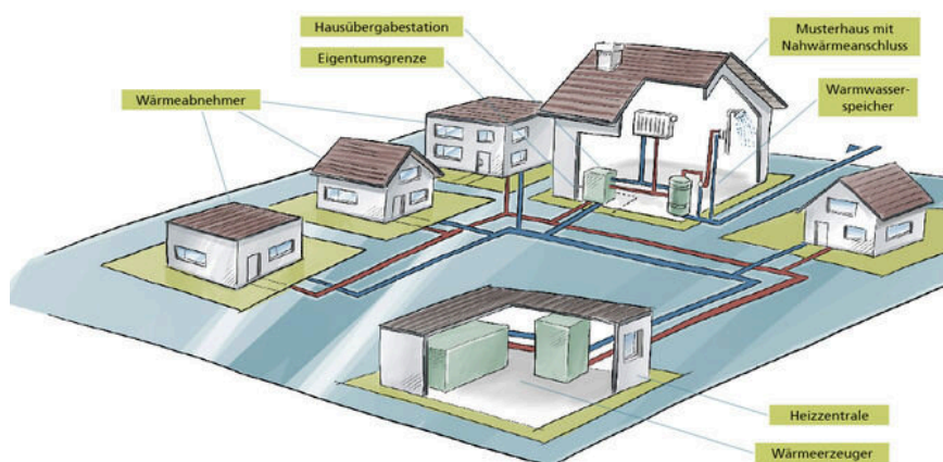
Schematische Darstellung eines Nahwärmenetzes. Quelle: Stadtwerke Pfronstetten
